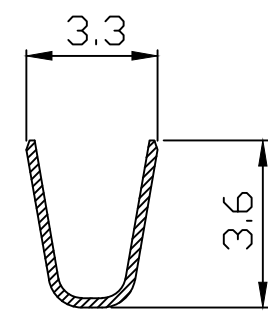
SEC A-A
