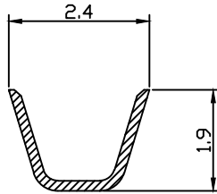
SEC A-A
