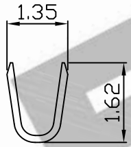
SEC A-A
